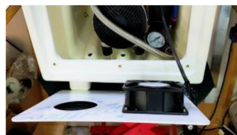
Ventilateur de refroidissement sur plaque amovible.
